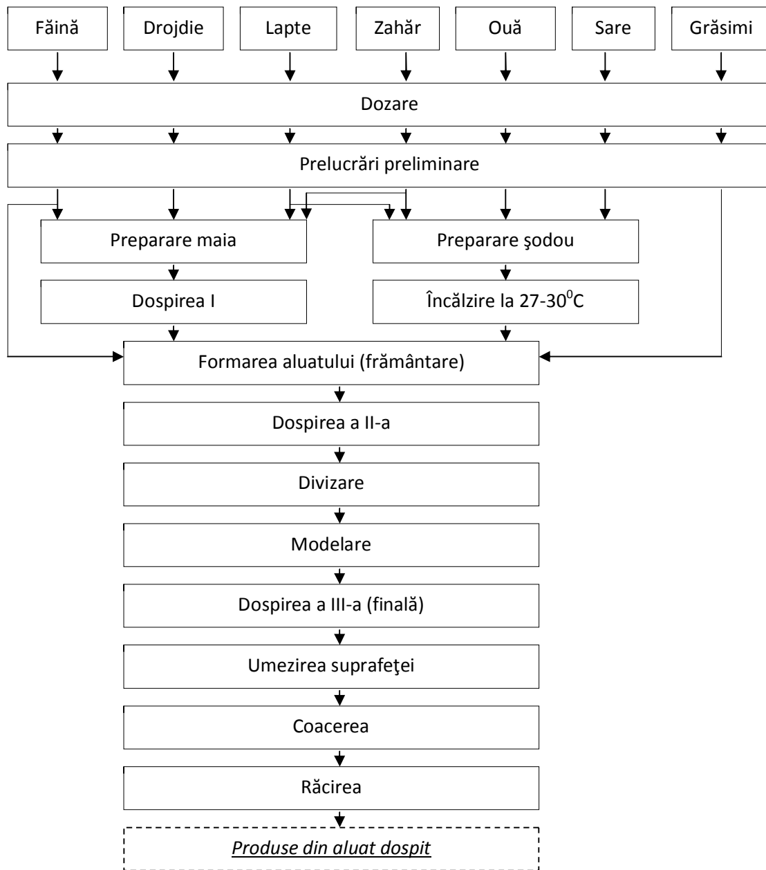
Fig.3.6.3. Schema tehnologică de obținere a preparatelor din aluat dospit (cu adaosuri) prin metoda indirectă
